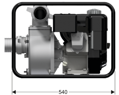
Dimensiones en milímetros
